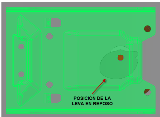
Figura 10: Leva posición Reposo
