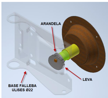
Figura 9: Montaje Leva y arandela
